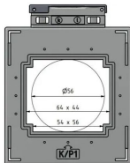
Masszeichnung-2
